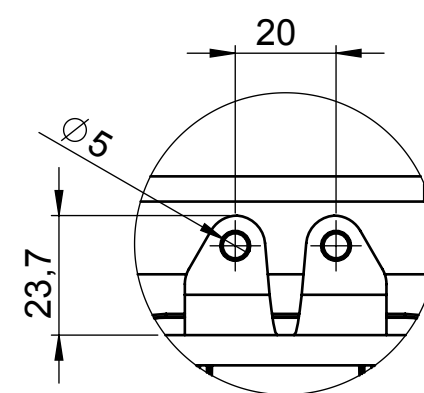
DETAIL A MAßSTAB 2 : 3
