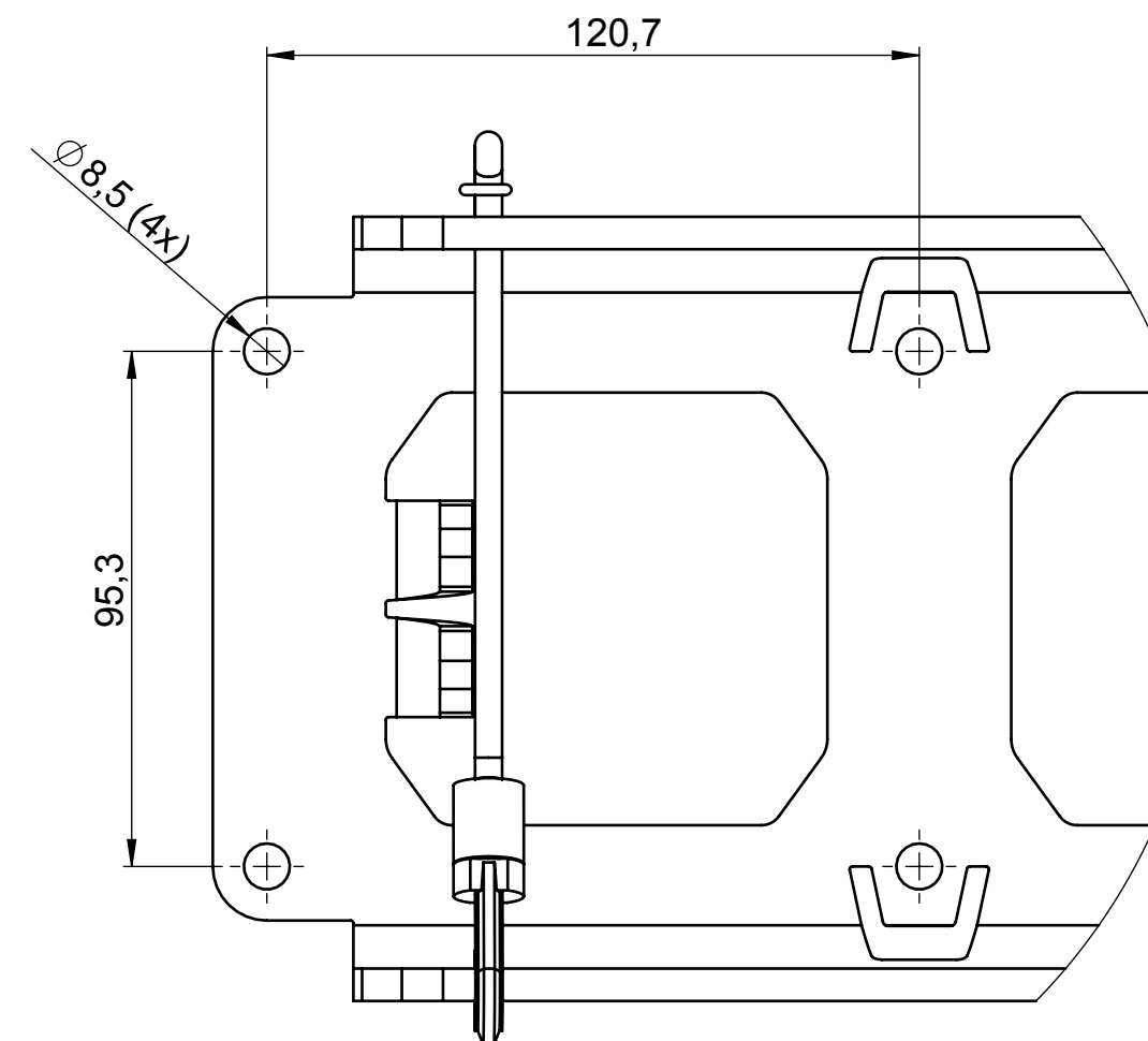
DETAIL B MAßSTAB 2 : 3
